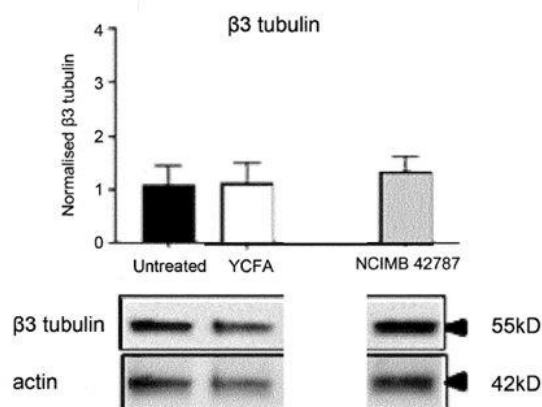
Слика 1B: Immunoblotting
