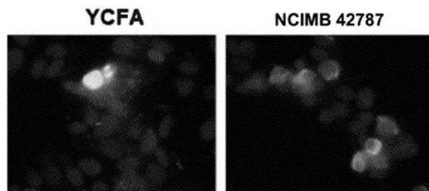
Слика 1: Level of \beta 3 Tubulin expression Слика 1A: Immunolabelling and cell imaging
