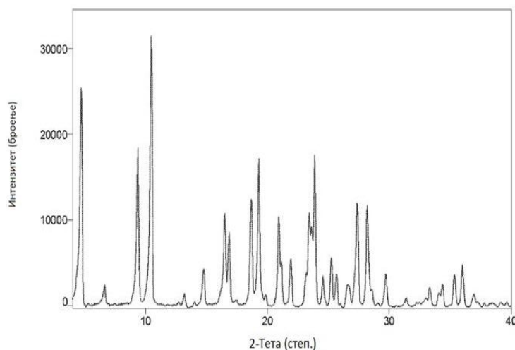
Шема на дифракција (XRPD) на рендгенски прав на соединение А, моно-HCl сол
