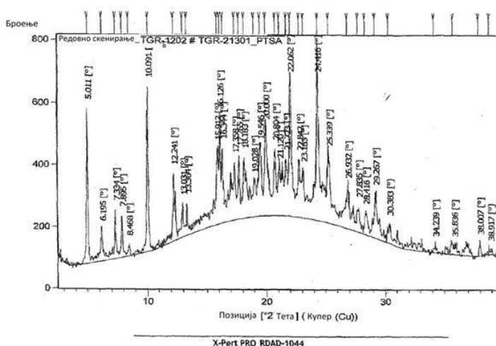
Слика 1: XRD СКЕНИРАЊЕ ЗА ПРИМЕР 1
