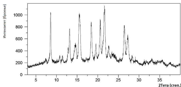
Слика 1: XRPD образец од форма 1
