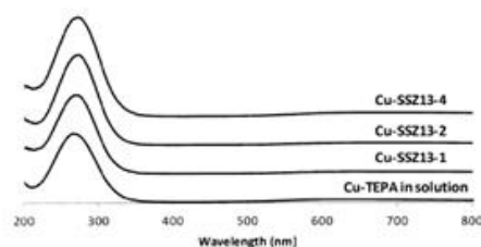
Слика 2 UV-Vis spectra of Cu-TEPA complex in solution and as-prepared Cu-SSZ-13 zeolites
