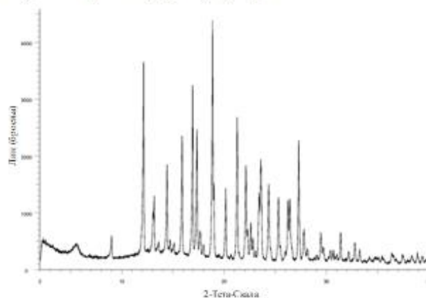
Нацрт 1 Слободен молекул (без сол) Пример 1 PXRD
