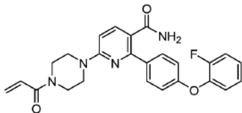
6-(4-акрилоилпиперазин-1-ил)-2-(2-флуоро-4-феноксифенил)никотинамид;
