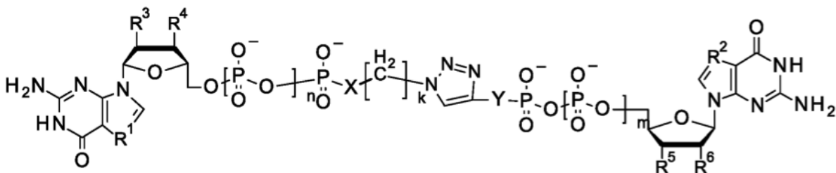
Формула I
