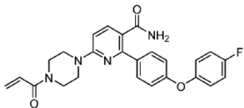
6-(4-акрилоилпиперазин-1-ил)-2-(4-(2-флуорофенокси)фенил)никотинамид;
