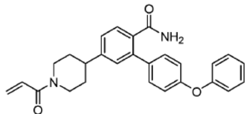
5-(1-акрилоилпиперидин-4-ил)-4'-феноксибифенил-2-карбоксамид;
