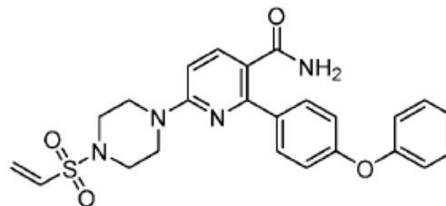
2-(4-феноксифенил)-6-(4-(винилсульфонил)пиперазин-1-ил)никотинамид;
