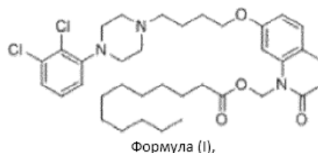
Формула (I),
