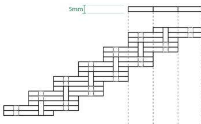
Слика 2 - Страничен преглед на поединечните модули и логика на спојување
