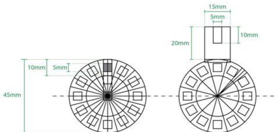
Слика 1 - Геометрија на хеликс составен од 12 дела за една цела ротација
