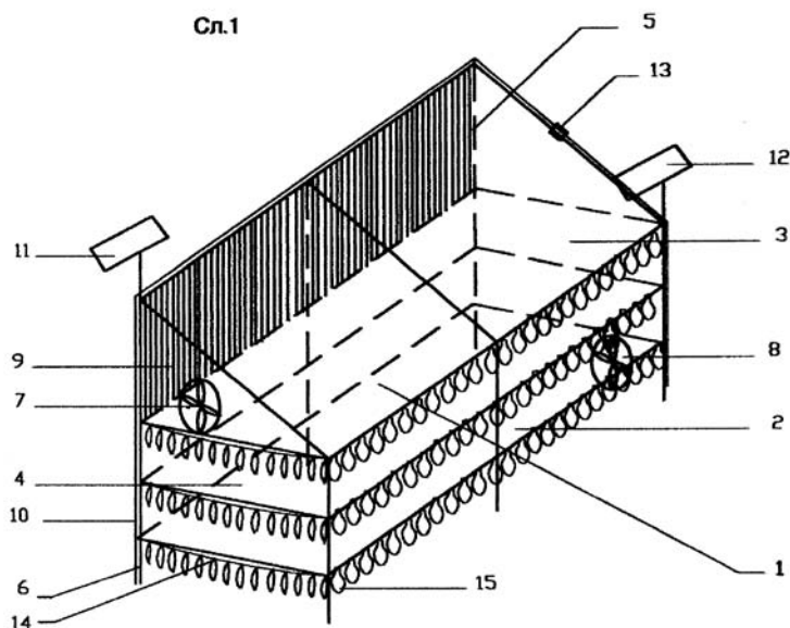
Соларна полиетиленска универзална сушница
