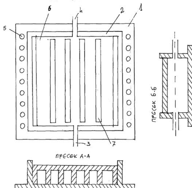
Слика бр. 1 Сончев колектор со директно загревање на водата - поглед одозгора
