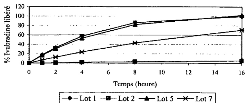
Слика 1: кинетика на растворање ин-витро Истиснувачи (екструдати) на хлорхидрат на ивабрадинот 10% + Eudragit 90% Вертикално: ослободен ивабрадин Хоризонтално: Време (часови)
