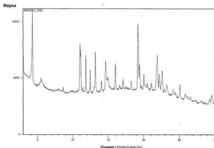
Нацрт 1: Дифрактограм RX на делта формата на периндоприл аргинин
