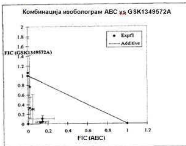
Слика 1: Инхибиција на ХИВ-1 RT од страна на соединение од формула (I), GSK1349572A, во комбинација со абакавир (ABC)
