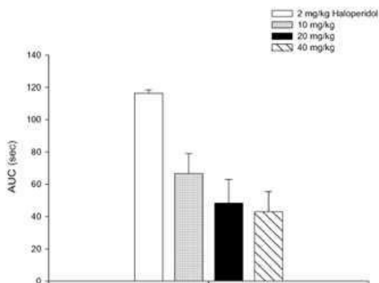
Слика 1: ST3932 ефикасност на антагонизирање на халоперидол-индуцирана каталепсија кај глушец
