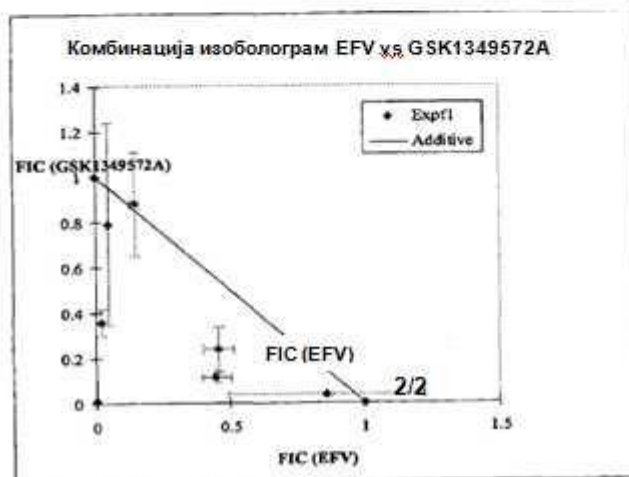
Слика 2: Инхибиција на ХИВ-1 RT од страна на соединение од формула (I), GSK1349572A, во комбинација со ефавиренц (EFV)
