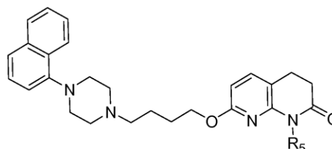
Формула (V)
