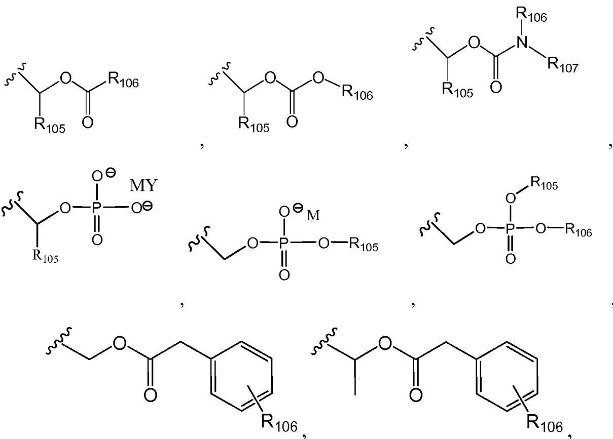
Формула (XIII)
