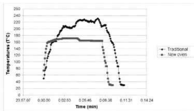
Сл. 1. Дијаграм на температури на печење
