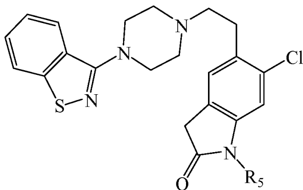
Формула (X)
