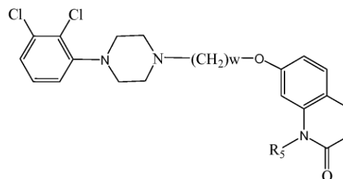
Формула (V)
