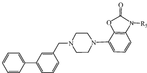
Формула (X)
