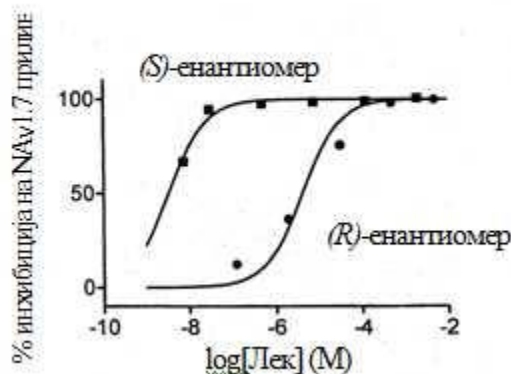
Стереоселективен блок од прилив на гванидинум во hNA v 1.7
