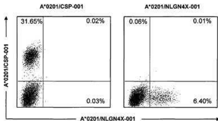
СЛИКА 1: Пример на in vitro имуногеницитет на IMA950 класа I TUMAP
