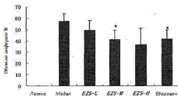
СЛИКА 1. Ефекти на аналгексинот врз обемот на церебрален инфаркт 48 часа по перманентен МСАО. Вредностите се изразени како процент од обемот (значи \pm SD) за 3 животни по група. Лажна: лажна група, Модел: модел група, Аналгексин-Л: аналгексин во мала доза; Аналгексин-М: аналгексин во средна доза; Аналгексин-Х: аналгексин во голема доза. * P<0.05 во споредба со модел групата.
