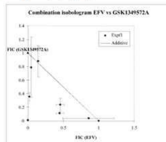
Слика 2: Инхибиција на HIV-1 iso со соединение со формула (I), GSK1349572A, во комбинација со ефавиренз (EFV)
