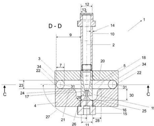
Нацрт 2
