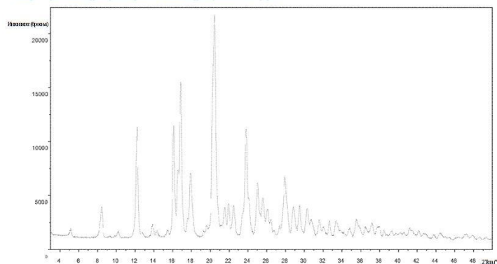
Фигура 1: Профил на дифракција на X-зраци. Модел на дифракција на ARN-509 форма В.
