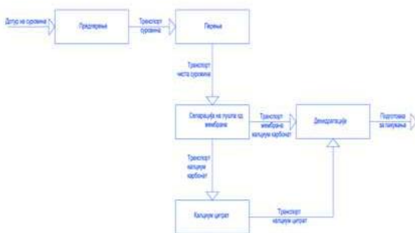
Слика 1 Функционална шема на технологија за преработка на лушпи од јајца
