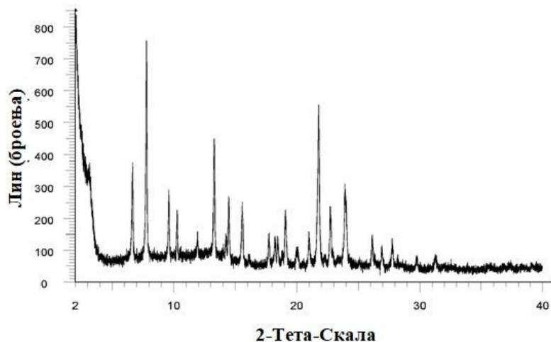
Нацрт 1: Модел на рендгенска прашковна дифракција на N-(2-{2-диметиламиноетил-метиламино}-4-метокси-5-{[4-(1-метилиндол-3-ил)пиримидин-2-ил]амино}фенил)проп-2-енамид форма А
