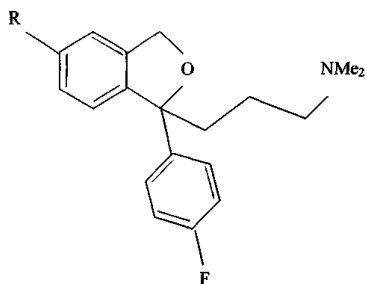
Формула (IV)
