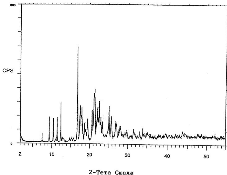
PXRD модел за P226
