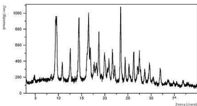
Слика 1: форма А на образец за дифракција на прашок со X-зраци
