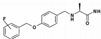
safinamide (Ia): 3-F
