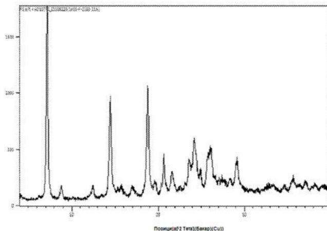
Сл. 1: XRD од форма I нилотиниб бензенсулфонат од пример 1.
