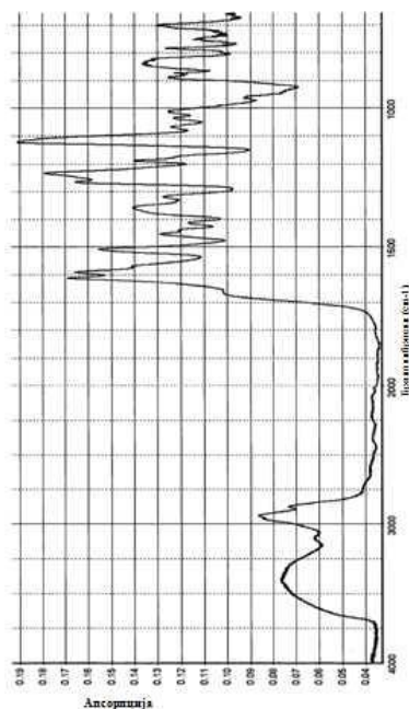
Напрг 1: Инфрацрвен спектар (микроATR) од ТМС435 На сол
