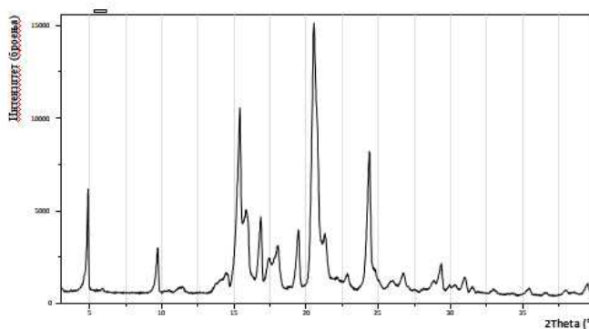
Напрат 1А: Форма А од слободна форма од соединение 1А
