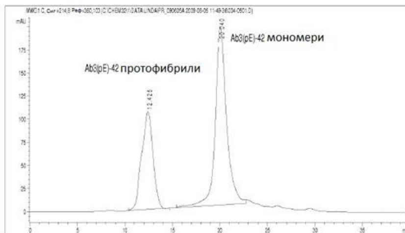
SEC-HPLC анализа на А \beta 3(pE)-42 протофибрили
