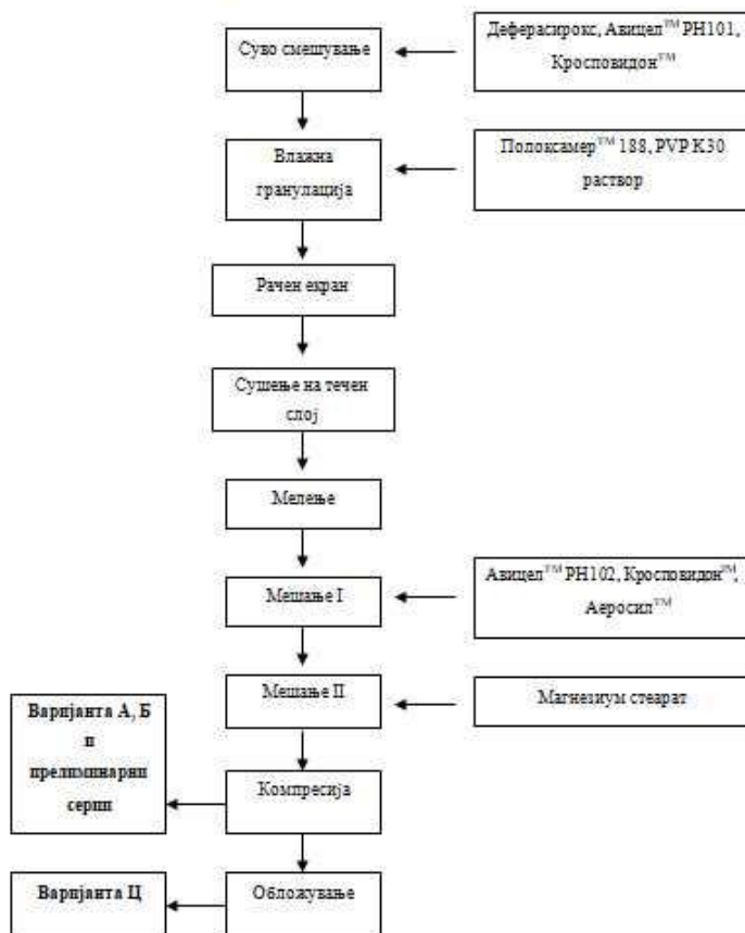
Нацрт 1: Процес на производство на обложени деферасироки таблети подготвени со влажна гранулација
