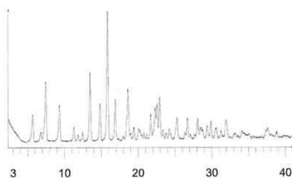
2-Тета-Скала
