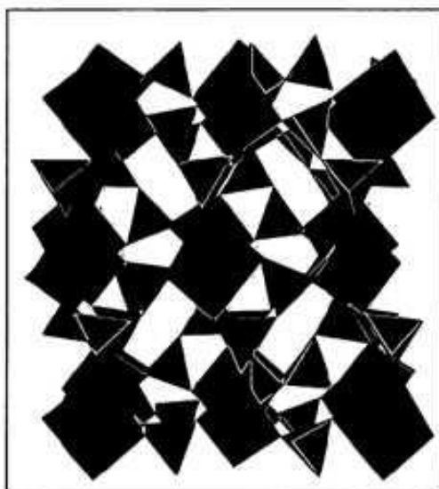
Темно=ZrO 3 (окт), Светло=SiO 2 (тет), катјони не се прикажани
