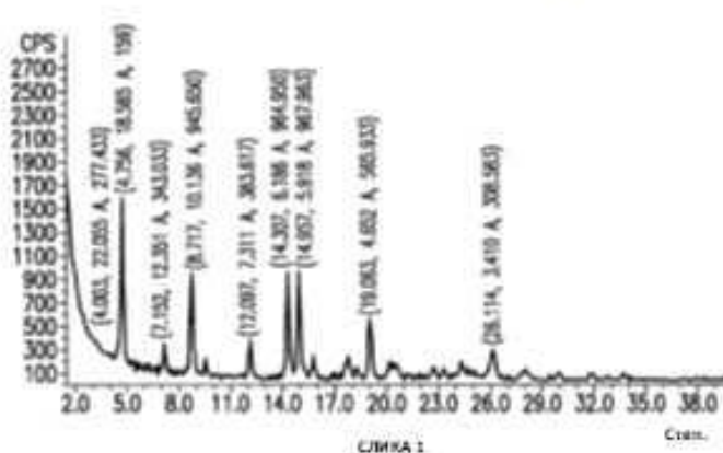
XRPD образец на хидрохлат на соединението (I-S)
