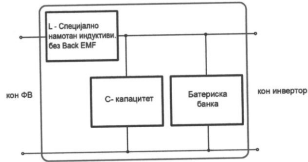
Сл.1 ПОДОБРУВАЊЕ НА ЕФИКАСНОСТА НА ФУНКЦИЈАТА НА ИНВЕРТОРИТЕ ЗА МРЕЖА "Maximum power point tracker" СОЛАРНИ ПАНЕЛИ КОРИСТЕЈЌИ „LC“ ЕЛЕМЕНТ СО ЕНЕРГЕТСКА БАНКА
