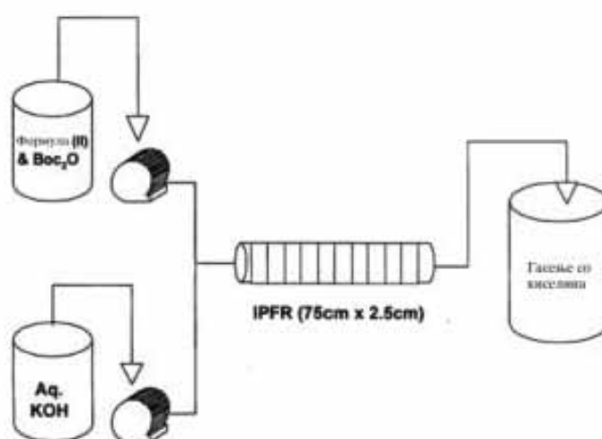
СЛИКА 1 Шематски приказ на IPFR
