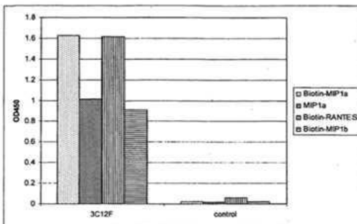
Нацрт 1 Поврзување на прочистен 3Ц12Ф со хемокин од ЕЛИСА.
