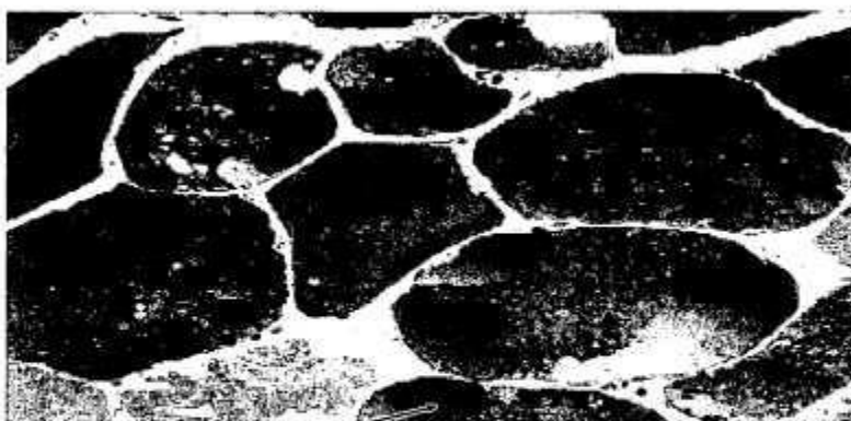
Слика 1. Светлиот микроскопски изглед на биопсија на скелетен мускул од пациент со GSD IIIa (MG). Пурпурно обоениот гликоген е присутен како цитоплазмички езера во миоцитите. Гликогенот не е ограден со мембрана во лизозомите, туку слободно тече во цитоплазмата.
