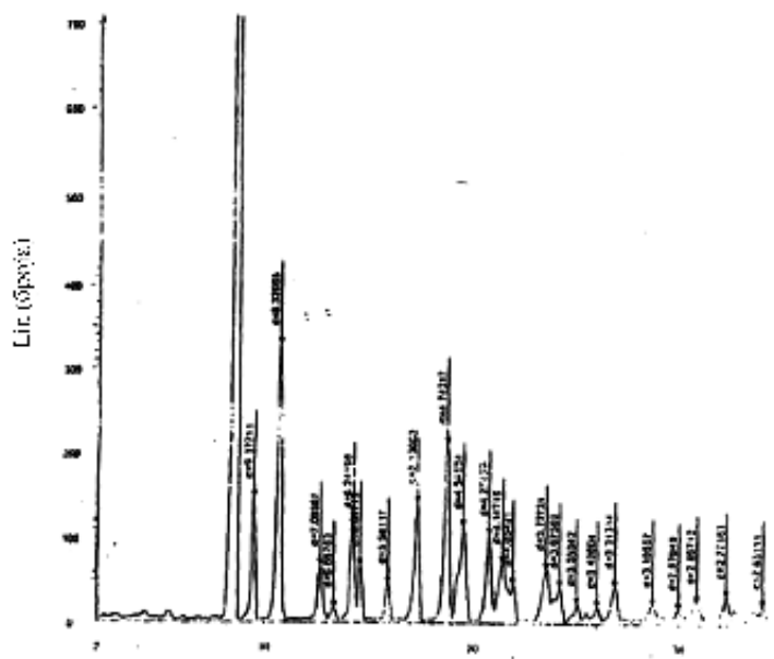
Слика 1: Модел на прекршување на X зраците врз прашок, на сол на периндоприл со дициклохексиламин.
