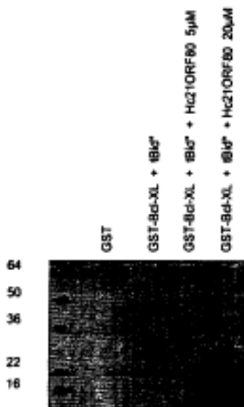
Сл. 1: "GST-одоојување" GST-Bcl-XL + Tbid со конкуренција на пептидот опишан со SEQ. ID. NO.1
