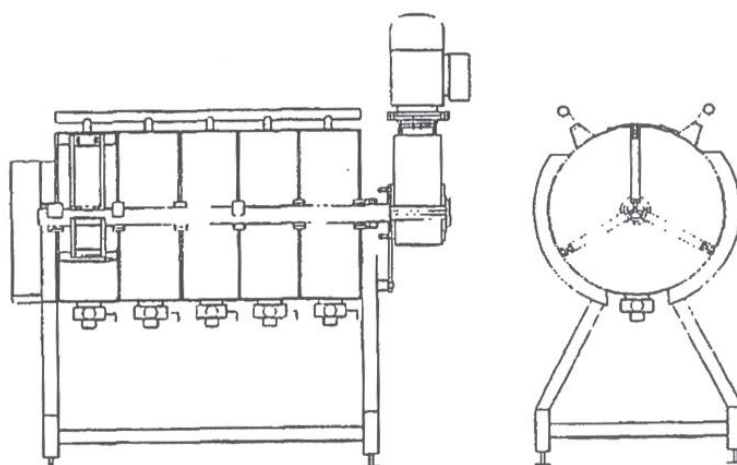
СЛИКА 1: Лонгитудинален поглед (лево) и попречен поглед (десно) на 5-коморниот реактор за хидролиза
