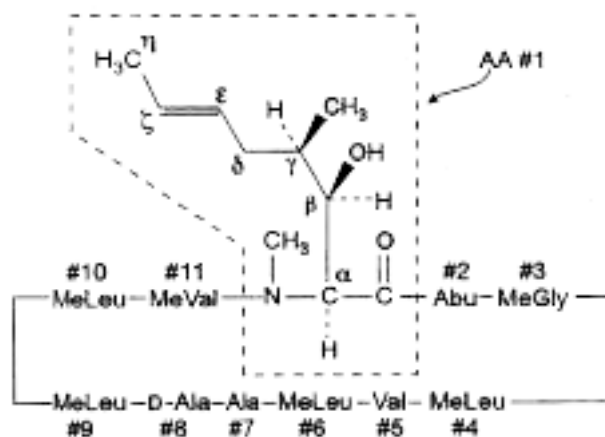
Циклоспорин-А
